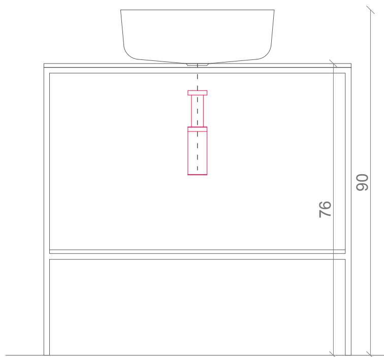
prospetto frontale
